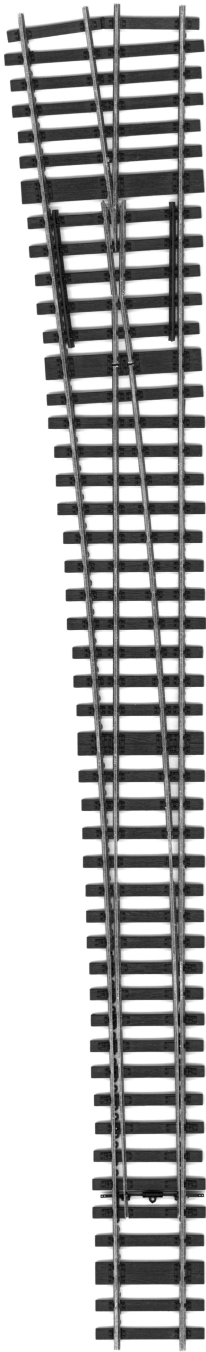
Linke Weiche 49-190-1:6,6 (8,6°) Bestellnummer 74661
